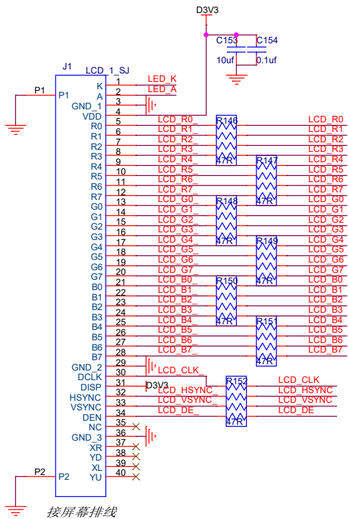
接屏幕排线
